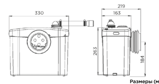
Размеры (мм)
